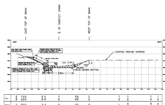
STA. 0+683.4
