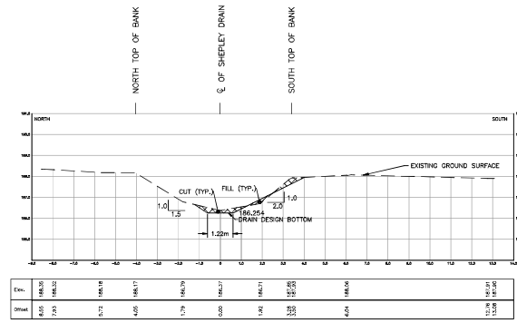
STA. 0+902.53
