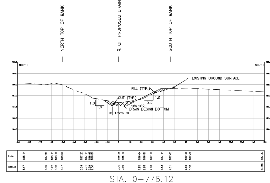
STA. 0+776.12
