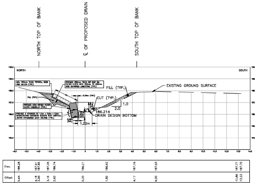
STA. 0+869.5
