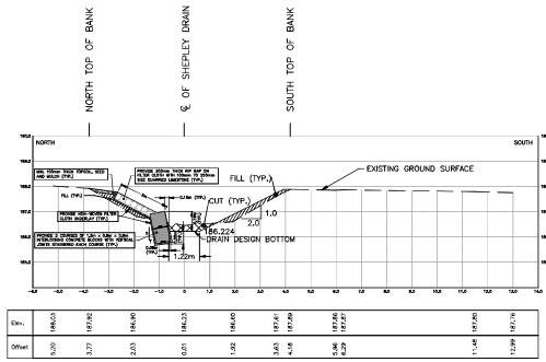
STA. 0+877.32
