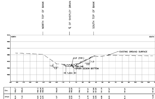
STA. 0+897.31
