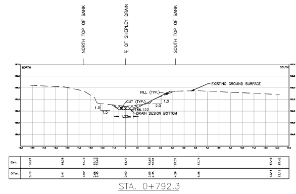
STA. 0+792.3
