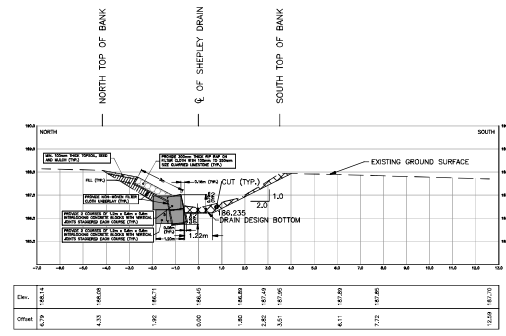
STA. 0+886.81
