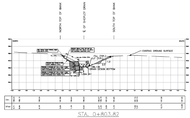
STA. 0+803.82
