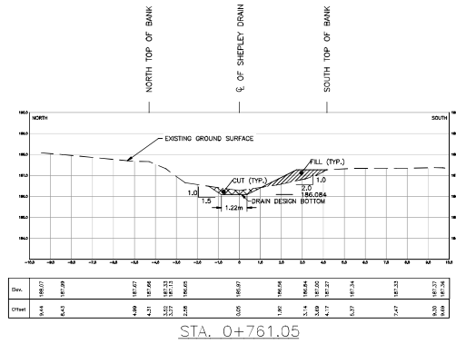
STA. 0+761.05
