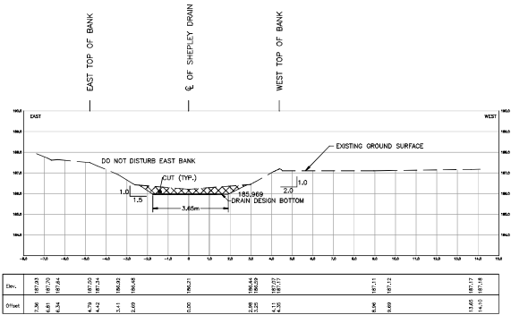
STA. 0+665.17
