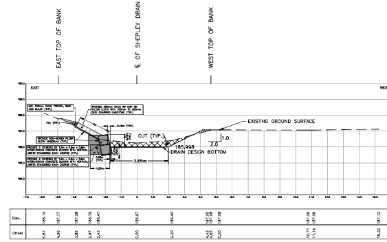
STA. 0+689.37
