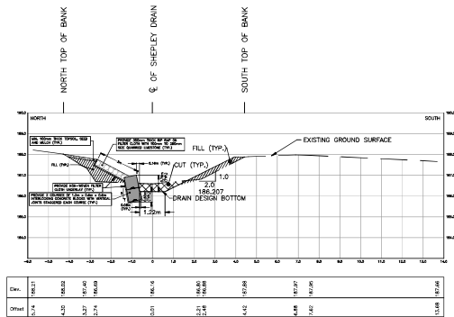
STA. 0+863.42
