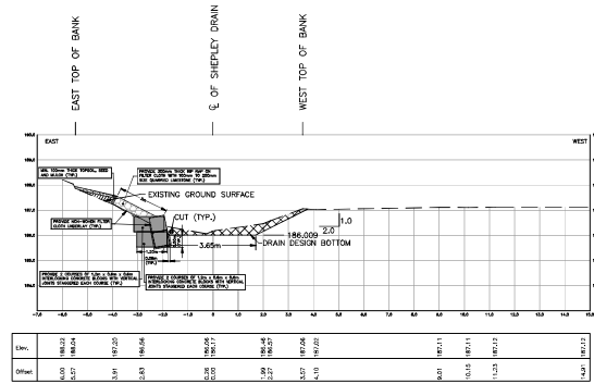
STA. 0+698.49
