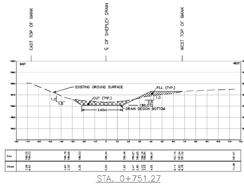
STA. 0+751.27
