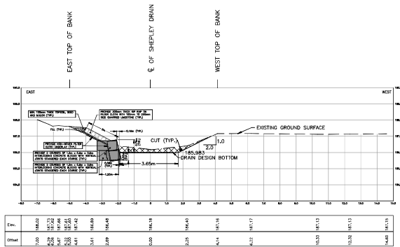
STA. 0+676.5
