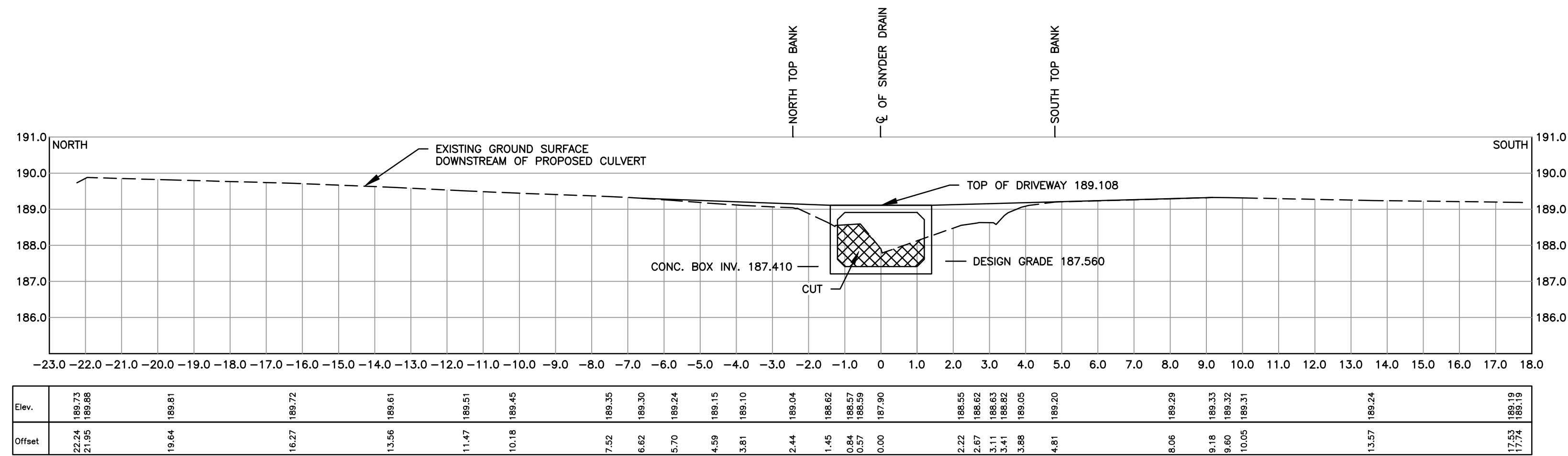
STA. 0+770.28 Scale = 1:100
