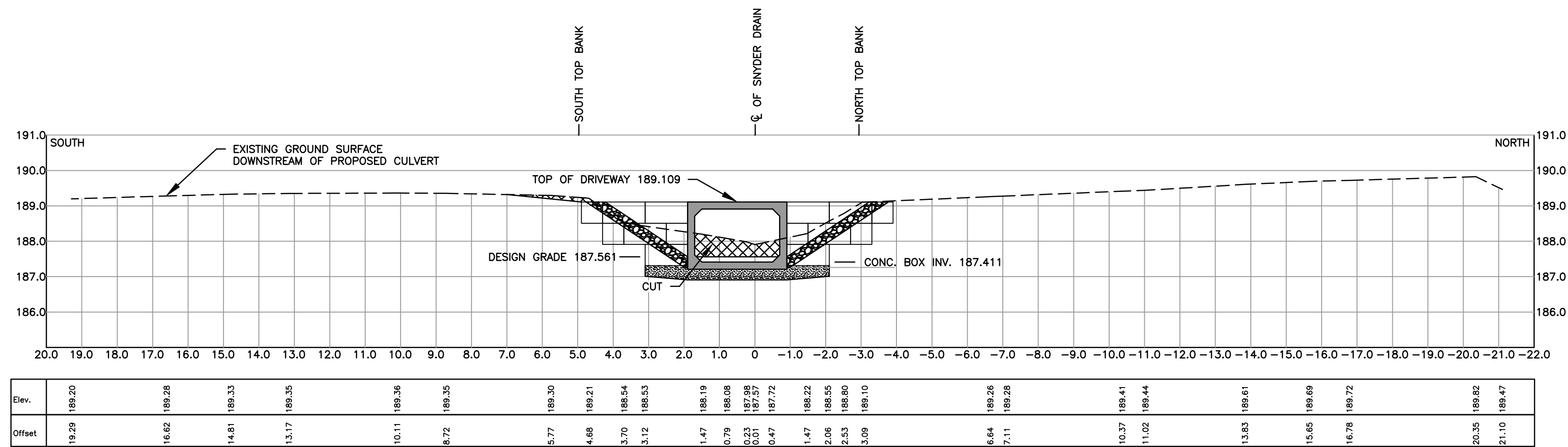
STA. 0+773.94 Scale = 1:100
