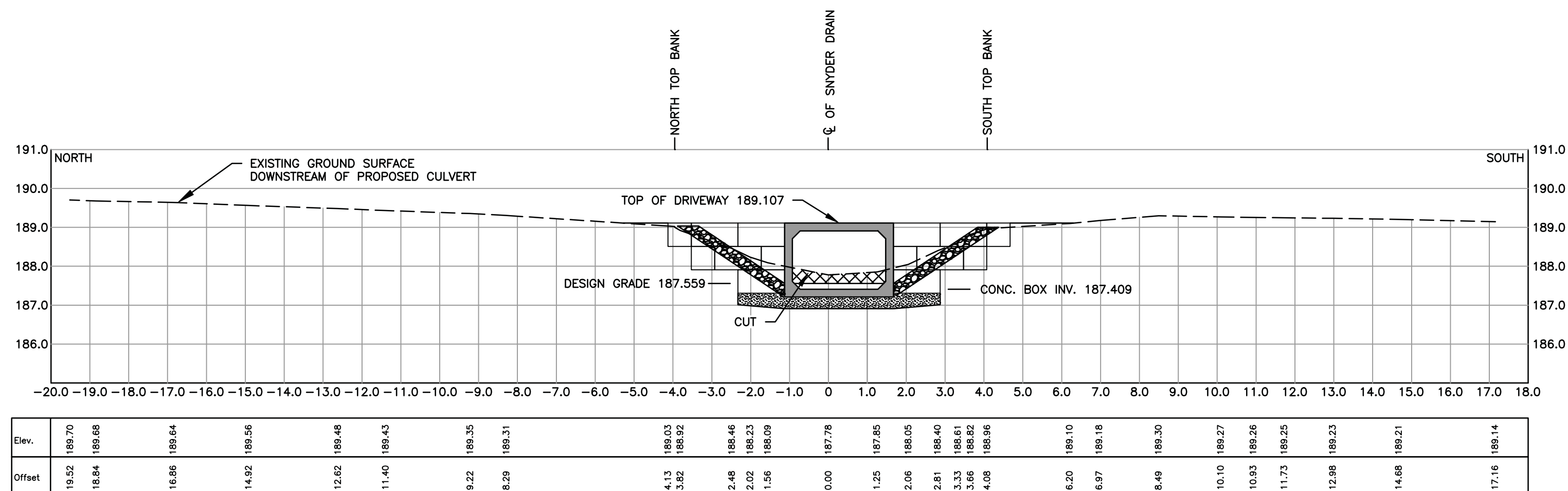
STA. 0+766.62 Scale = 1:100
