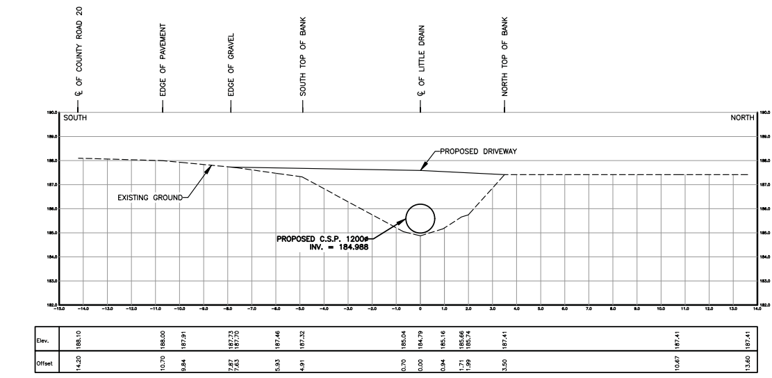
STA. 0+325.6 SCALE=1:100
