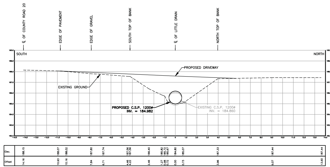
STA. 0+317.59 SCALE=1:100
