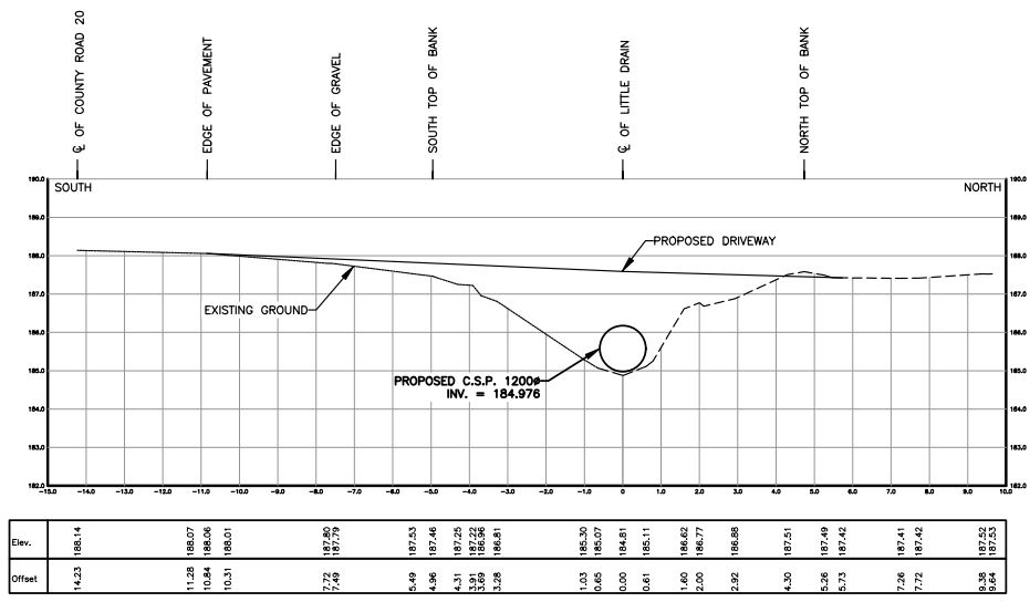
STA. 0+309.6 SCALE=1:100
